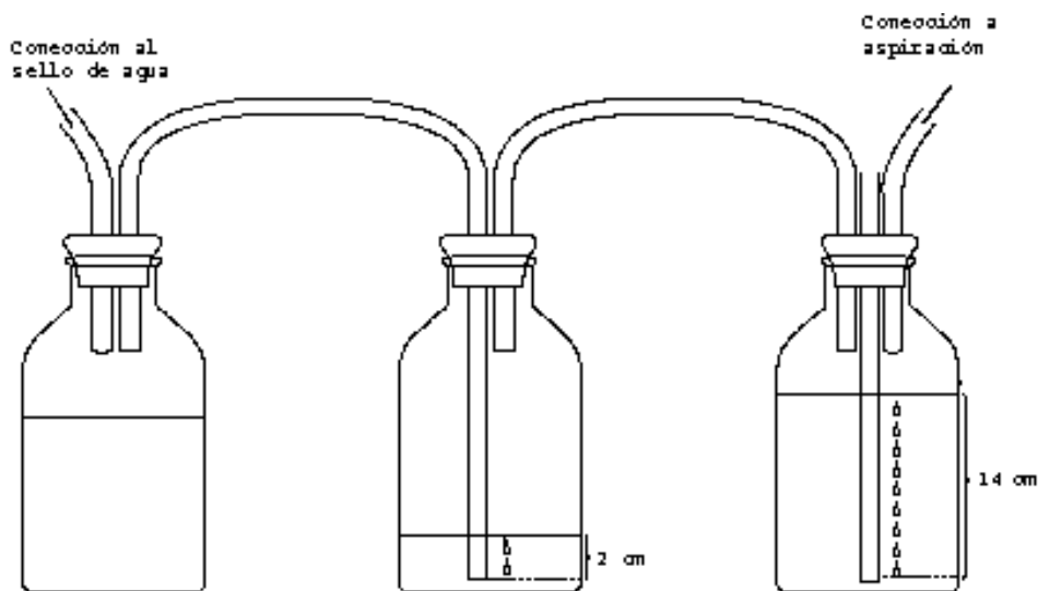
Figura 249: Sistema de aspiración con 3 frascos.
